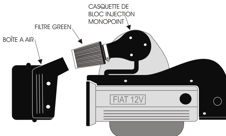
MONTAGE AVEC LE KIT ADMISSION GREEN
