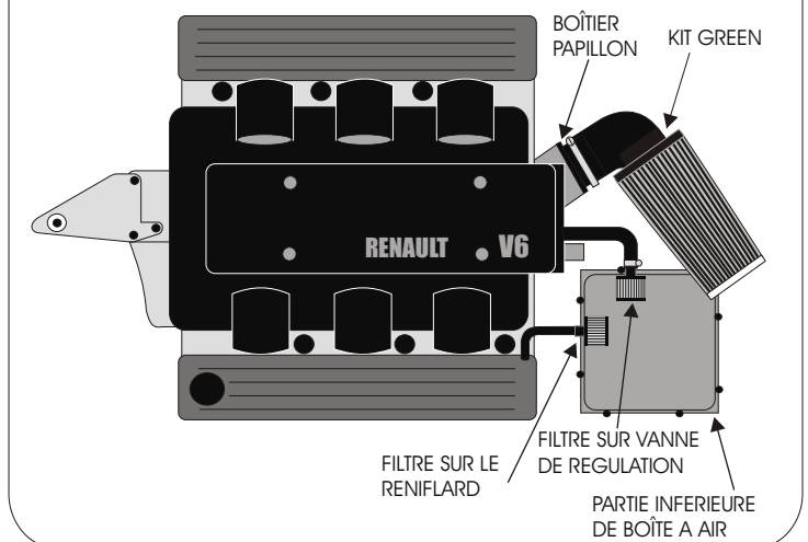
MONTAGE AVEC LE KIT ADMISSION GREEN
